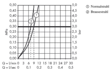
Durchflussdiagramm
